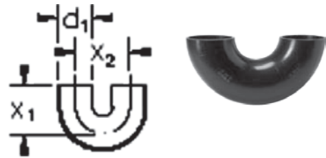
U-bend 180°
